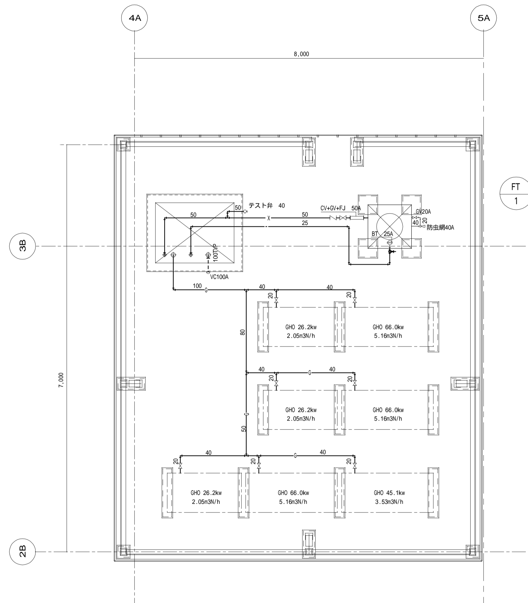
屋上機械置場詳細図(普通教室側)
